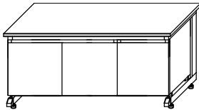
边台1200*800*600 (免疫室)
