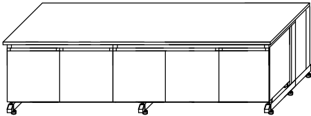
边台2400*1000*600 (生化室)
